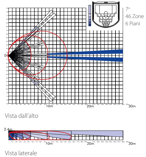
Lente: KX30-LR
